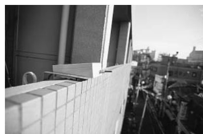
ワイヤレスインターネットマンションで用いる無線LAN。屋上に親機を設置し、各部屋のベランダに設置した子機と通信する。
