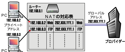
図3 NAT機能の仕組み
