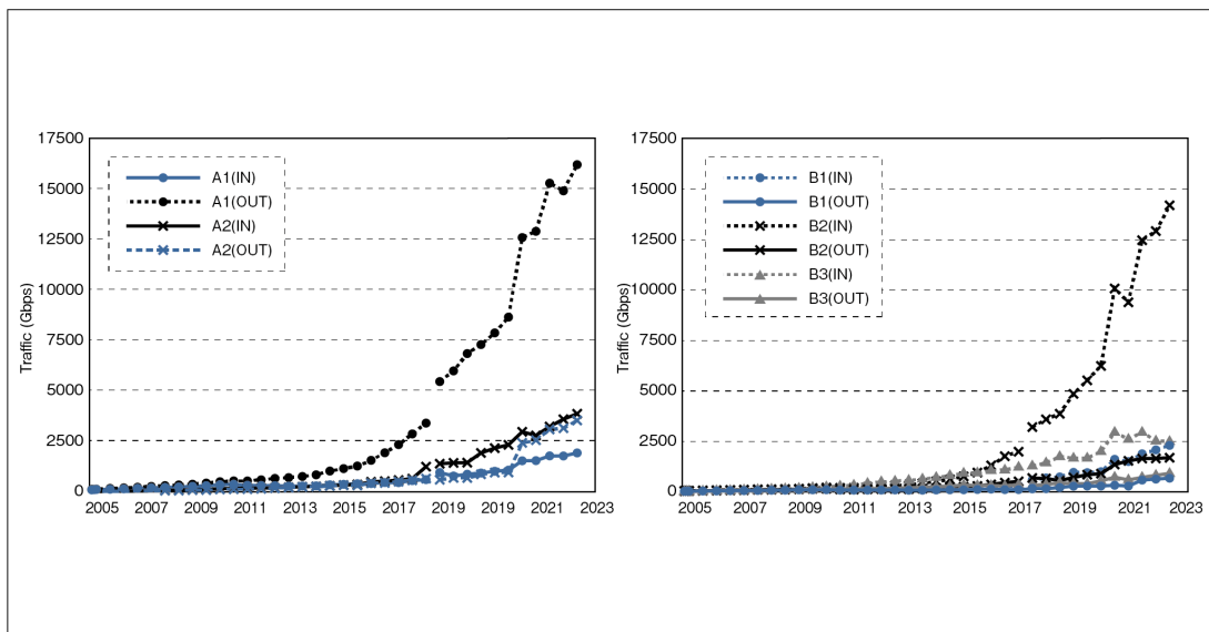
資料4-2-9 トラフィックの増加傾向：カスタマーtraフィック（左）と外部traフィック（右）
