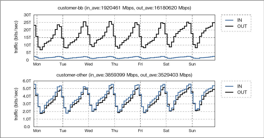
資料 4-2-6 2022 年 5 月の週間カスタマートラフィック：ブロードバンドカスタマー（上）とブロードバンド以外のカスタマー（下）
