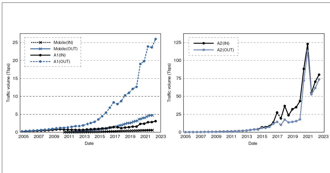
資料4-2-11 ブロードバンドカスタマー（左）およびブロードバンド以外のカスタマー（右）の総量推計値の推移
